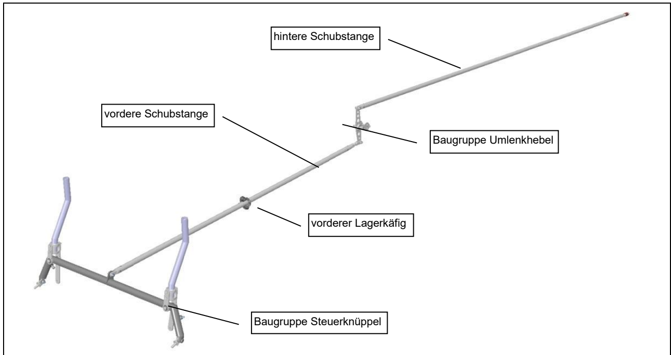
Übersicht Höhenrudersteuerung
